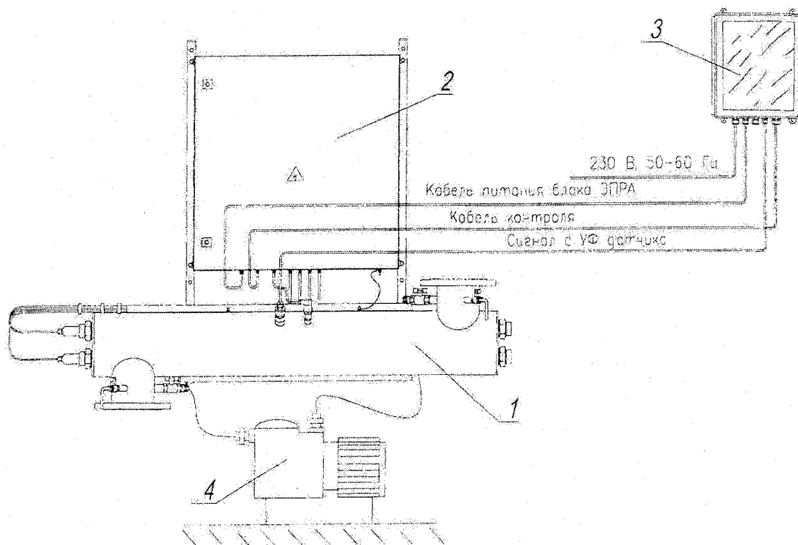
3. ábra. Az UV-besugárzással működő vízfertőtlenítő berendezés: 1 – fertőtlenítő kamra; 2 – EPRA blokk; 3 – kezelőpult; 4 – mosószivattyú.
